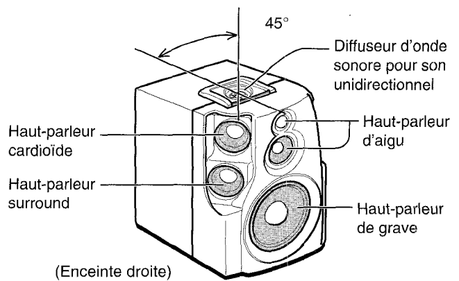
Figure 1 Enceinte acoustique à diffusion sonore frontale sur 180°
